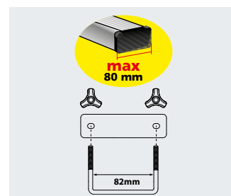
Kit di fissaggio Fixing kit
